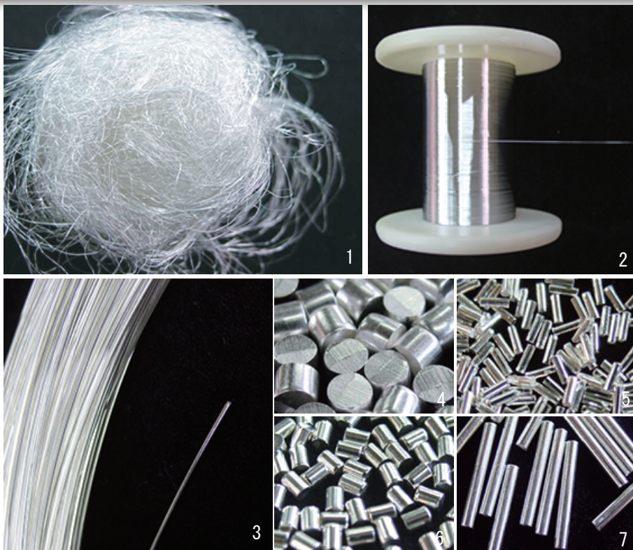
1. φ0.05mm 2. φ0.05mm (コイル巻き) 3. φ0.7mm 4. φ4×3mm 5. φ1×4mm 6. φ2×4mm 7. φ2×8mm
